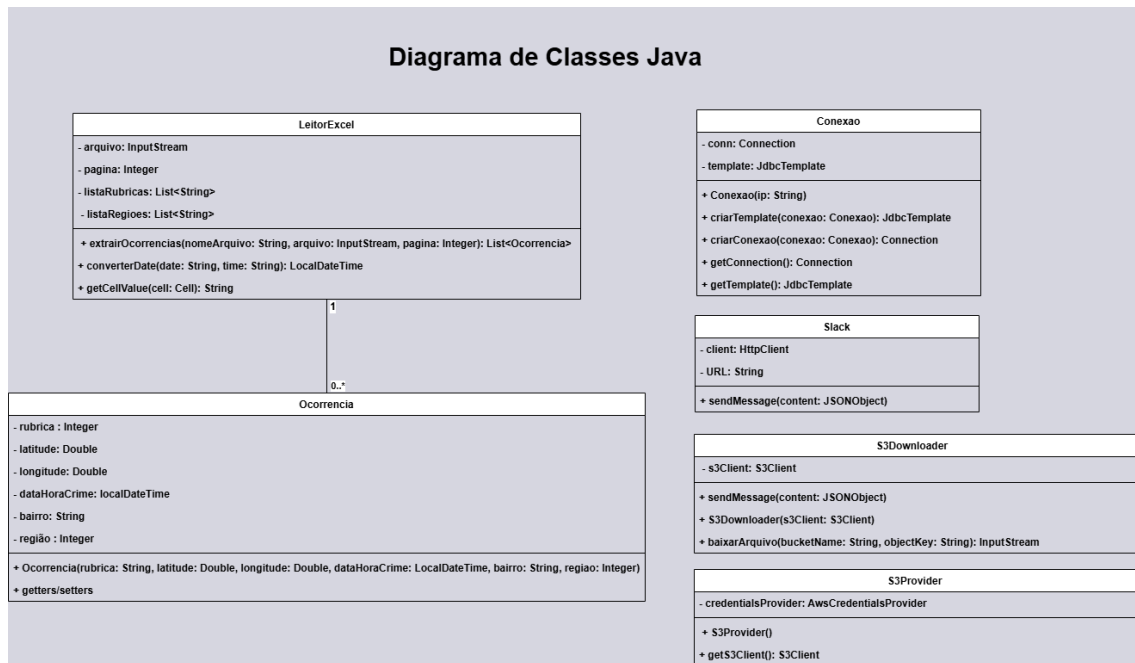
Figura 17 - Diagrama de Classes Java
