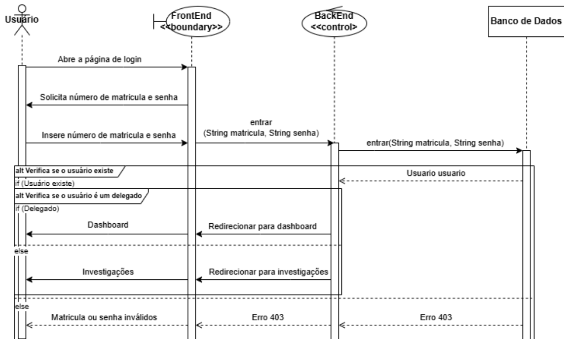
Figura 19 - Diagrama de Sequência Login
