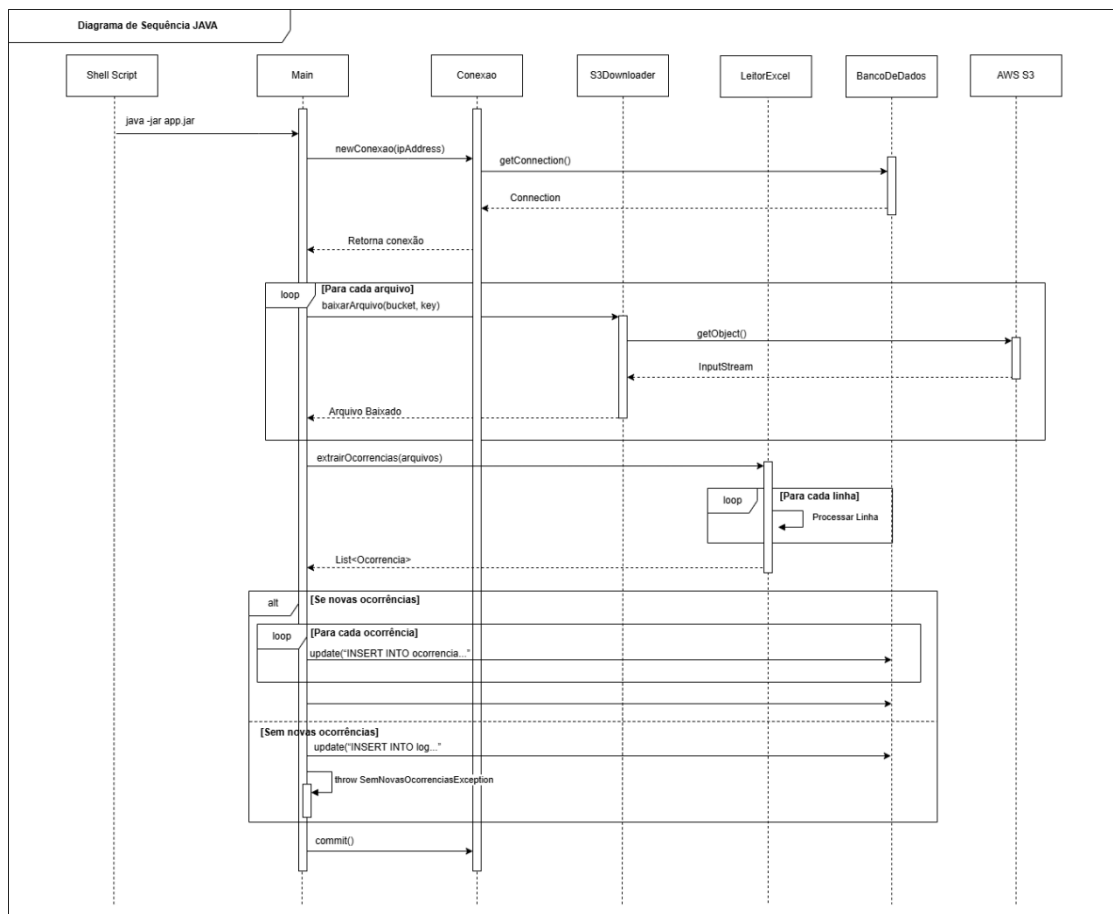
Figura 20 - Diagrama de Sequência Java
