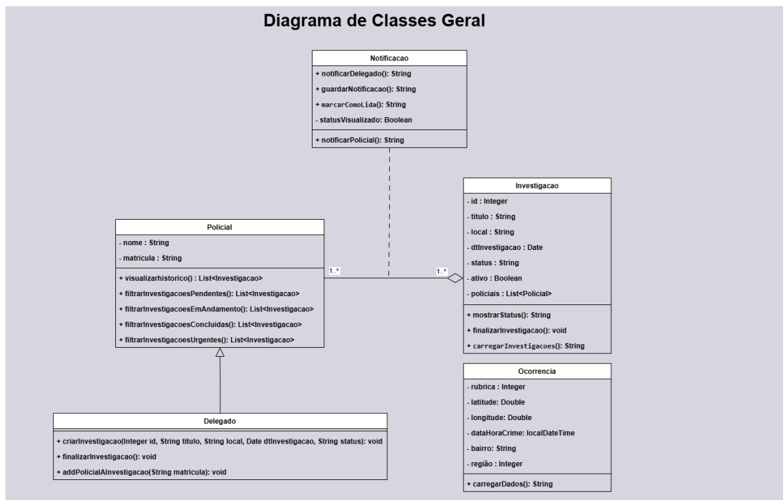
Figura 18 - Diagrama de Classes Geral do Sistema
